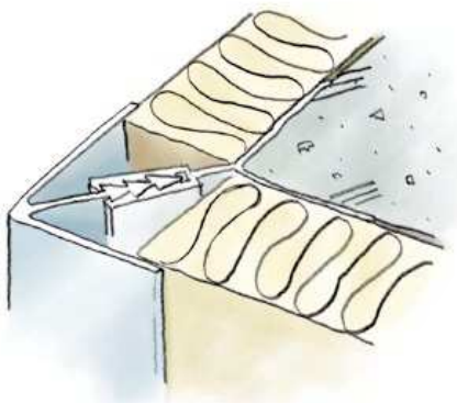
51135 アルミ AMD-25 (出隅カバー 25 mm用) 2.73m / アルマイトシルバー
