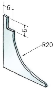
79054 アルミ CRS-2 サイドキャップ アルマイトシルバー/t=1.0mm
