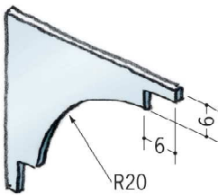
79053 アルミ CRS-1 サイドキャップ アルマイトシルバー/t=1.0mm
