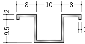
53088 アルミハット9.5×10 3m/アルマイトシルバー
