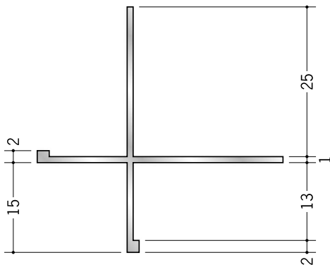
53170 アルミ XA-13+2 2.73m/アルマイトシルバー
