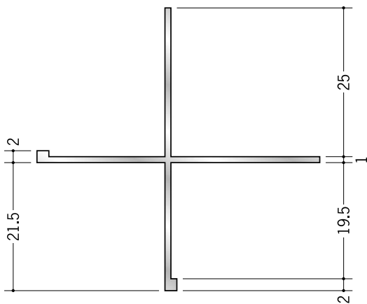
53152 アルミ XA-19.5+2 2.73m/アルマイトシルバー
