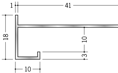
52317 アルミDTK-10 3m/アルマイトシルバー
