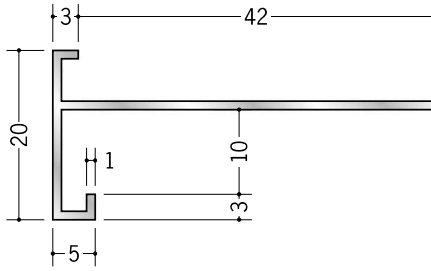
52117 アルミD型83 3m/アルマイトシルバー
