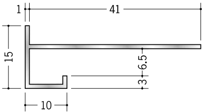
52315 アルミDTK-7 3m/アルマイトシルバー
