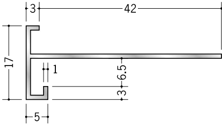
52115 アルミD型81 3m/アルマイトシルバー
