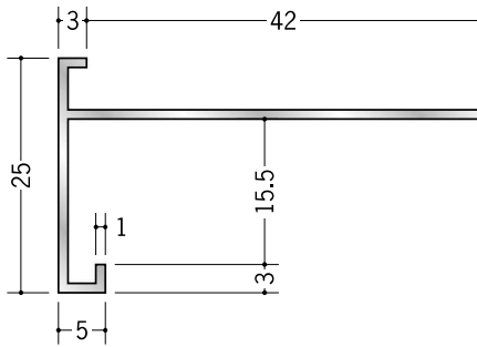
52119 アルミD型85 3m/アルマイトシルバー
