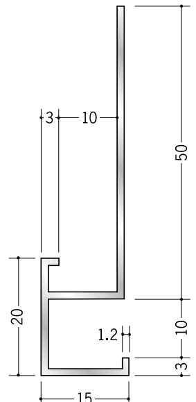
52092 アルミD型22 3m/アルマイトシルバー
