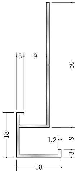
52094 アルミD型24 3m/アルマイトシルバー
