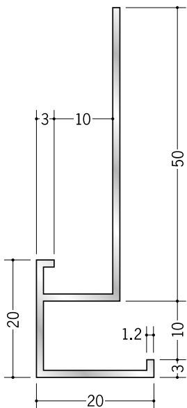
52102 アルミD型51 3m/アルマイトシルバー
