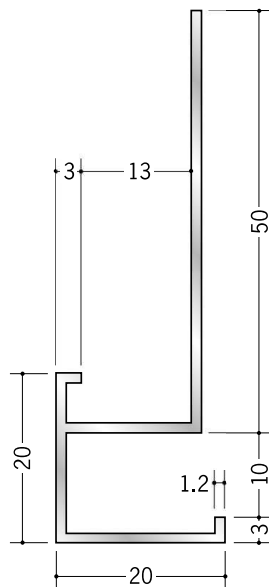
52097 アルミD型28 3m/アルマイトシルバー
