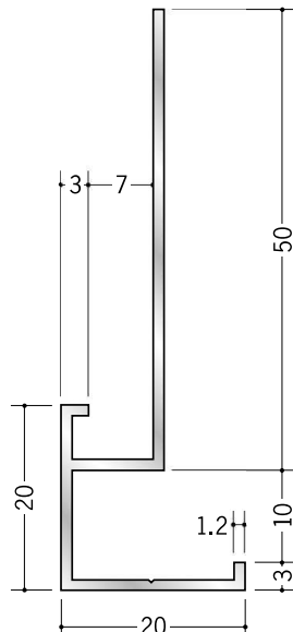
52101 アルミD型50 3m/アルマイトシルバー
