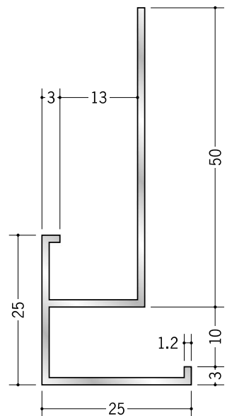
52109 アルミD型58 3m/アルマイトシルバー
