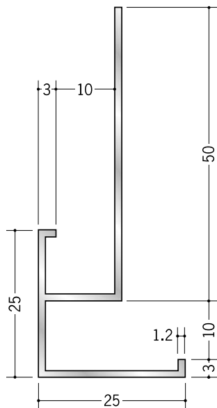
52108 アルミD型56 3m/アルマイトシルバー
