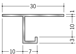
54002 アルミCSM-10 3m/アルマイトシルバー
