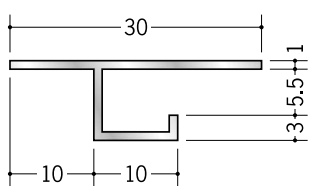
52255 アルミCS-1005 3m/アルマイトシルバー
