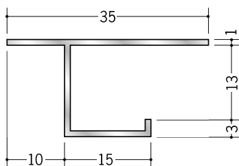
52154 アルミB型1012 3m/アルマイトシルバー
