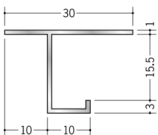
52256 アルミCS-1015 3m/アルマイトシルバー
