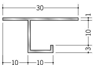
52053 アルミCS-1009 3m/アルマイトシルバー
