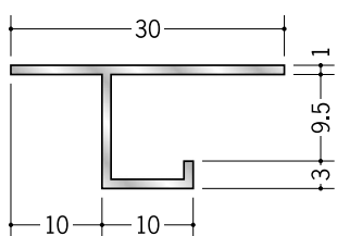
53225 アルミCS-岩綿9 3m/アルマイトシルバー
