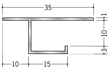
52153 アルミB型1009 3m/アルマイトシルバー
