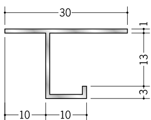
52054 アルミCS-1012 3m/アルマイトシルバー
