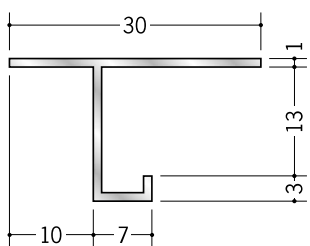
54003 アルミCSM-13 3m/アルマイトシルバー
