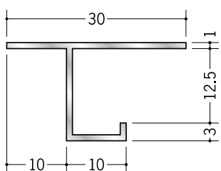
53226 アルミCS-岩綿12 3m/アルマイトシルバー
