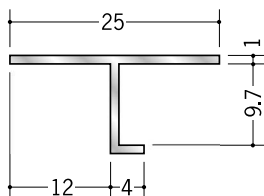
50002 アルミ ATV-1209 3m/アルマイトシルバー
