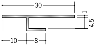
50053 アルミ ATE-4 3m/アルマイトシルバー
