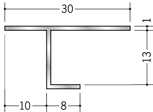
50070 アルミ ATE-13 3m/アルマイトシルバー
