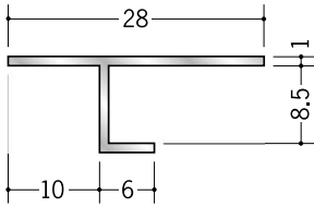
50224 アルミ ATS-8 3m/アルマイトシルバー
