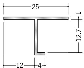
50003 アルミ ATV-1212 3m/アルマイトシルバー
