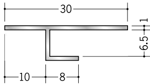
50054 アルミ ATE-6 3m/アルマイトシルバー
