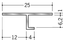
50001 アルミ ATV-1206 3m/アルマイトシルバー
