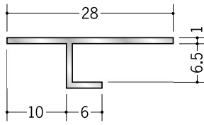
50223 アルミ ATS-6 3m/アルマイトシルバー
