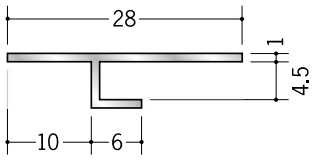
50221 アルミ ATS-4 3m/アルマイトシルバー
