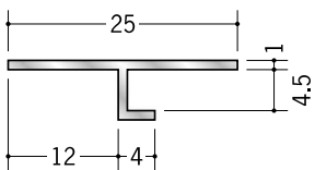
50004 アルミ ATV-1204 3m/アルマイトシルバー
