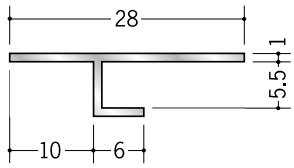
50222 アルミ ATS-5 3m/アルマイトシルバー
