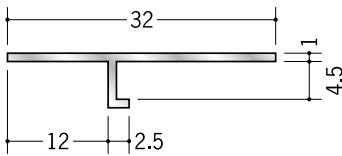
50045 アルミ AT-4 3m/アルマイトシルバー
