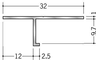
50051 アルミ AT-9 3m/アルマイトシルバー
