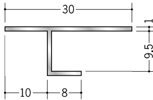
50055 アルミ ATE-9 3m/アルマイトシルバー
