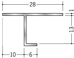
50226 アルミ ATS-12 3m/アルマイトシルバー
