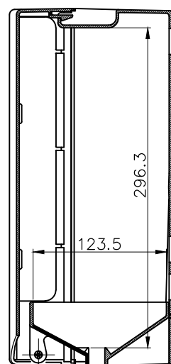
A-A断面図
