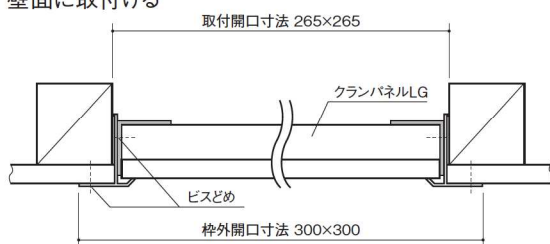
■取付図
