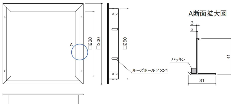
■仕様図
