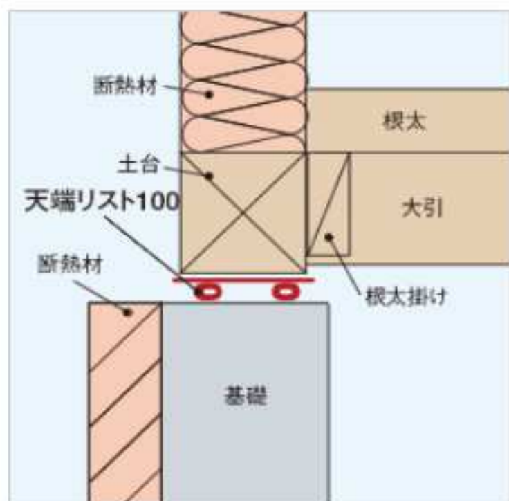
天端リスト100・500納まり断面図。
