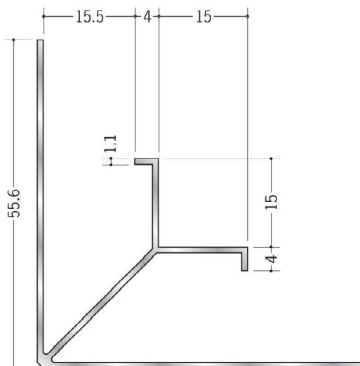
59069 アルミ入隅15型 アクリル焼付 3m/ネオシルバー・ネオステンカラー
