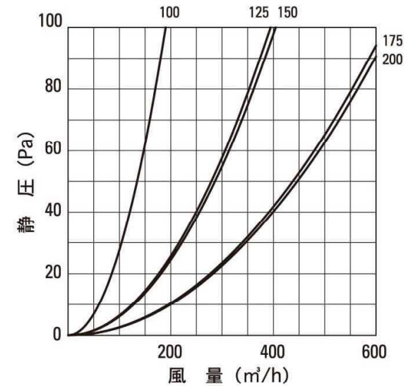
圧力損失曲線
