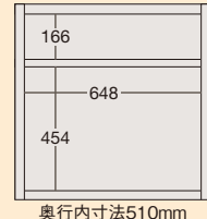
モニター収納部内寸法図
