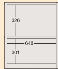
周辺機器収納部内寸法図
