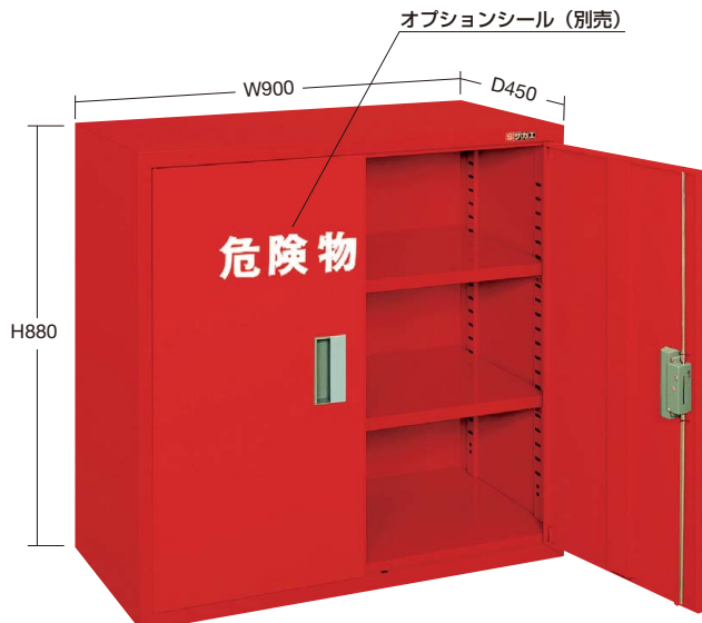
KU-AR ●棚板寸法：W875×D400×H25mm
