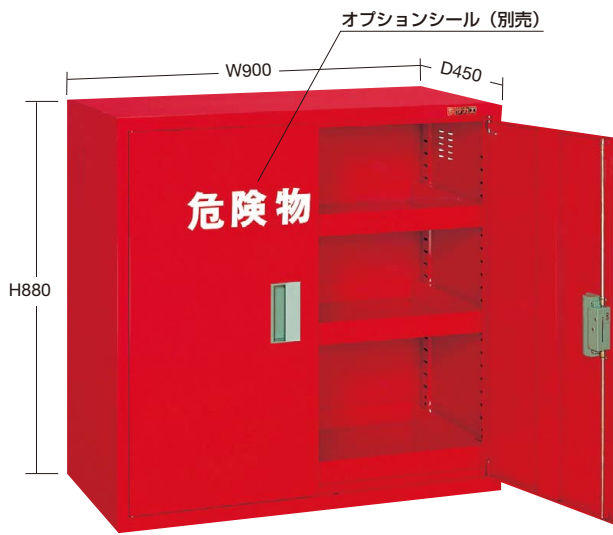
KU-AR1 (通気孔有り) ●棚板寸法：W845×D400×H48mm
