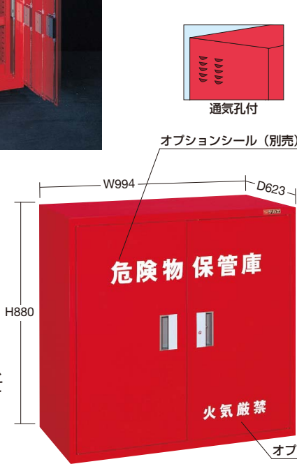
KU-KAR1 (通気孔有り) ●棚板寸法: W805×D555×H48mm
