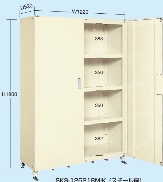
SKS-125218MIK (スチール扉)
