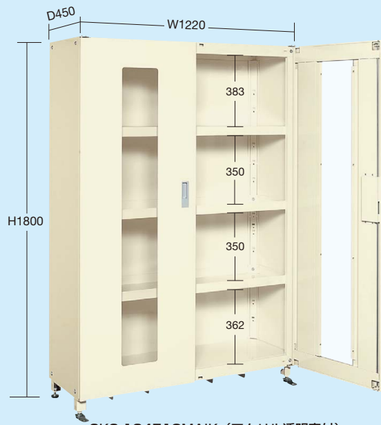
SKS-124518MAIK (アクリル透明窓付)
