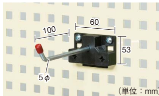
(単位: mm)
