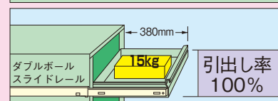
NKL-95JI (単位: mm)
