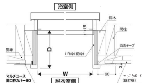
■マルチユース開口枠カバー60納まり図
