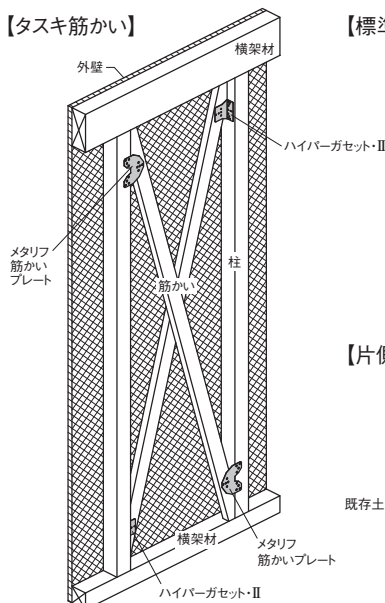
■取付図
