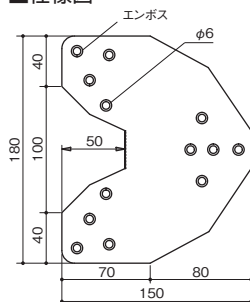
■仕様図
