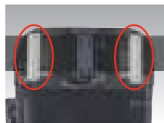
ベルトからの浮きを防止するサイドクリップ (SFKBN-2Mのみ)
