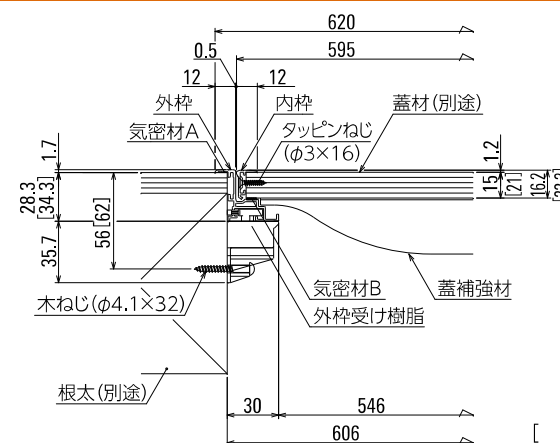
納まり図
