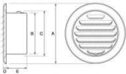
寸法図
