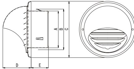
■ 寸法図
