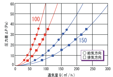
■ 通気量試験表
