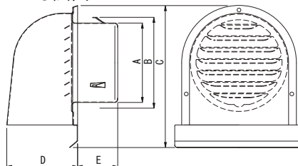
■ 寸法図
