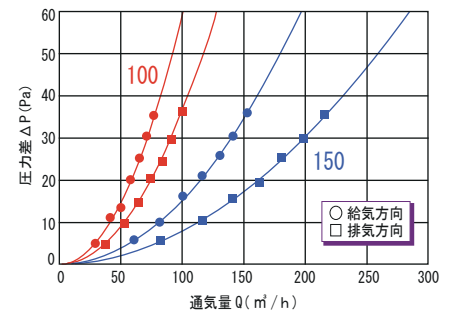
■ 通気量試験表
