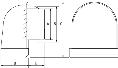
■ 寸法図
