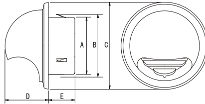
■ 寸法図
