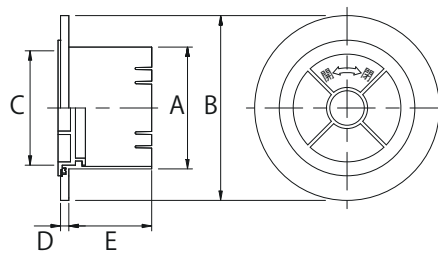
■寸法図
