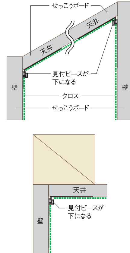
参考納まり図(天井一壁)
