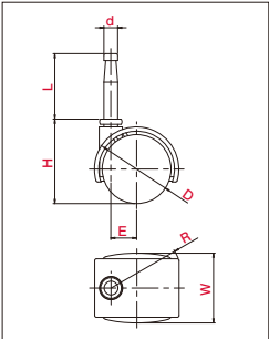
・図面〔差し込み式〕
