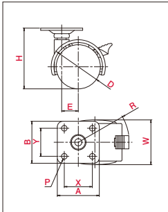
・図面〔プレート式ストッパー付〕
