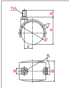
・図面〔ねじ込み式ストッパー付〕
