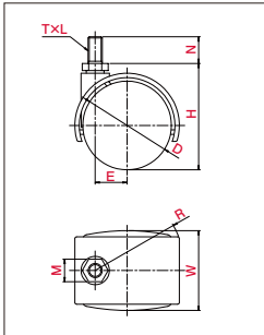
・図面〔ねじ込み式〕
