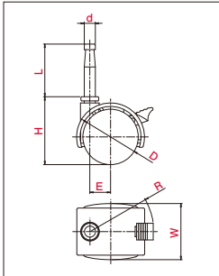
・図面〔差し込み式ストッパー付〕
