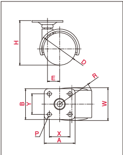
・図面〔プレート式〕
