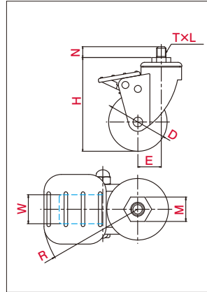
樹脂キャスターφ75, M12×14
