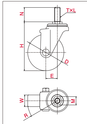
SUS-SJT-100N, M20×40
