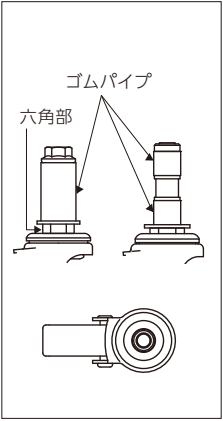
・取付方法〔差し込み式〕
