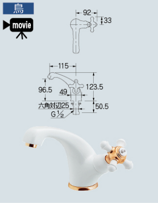
立水栓
