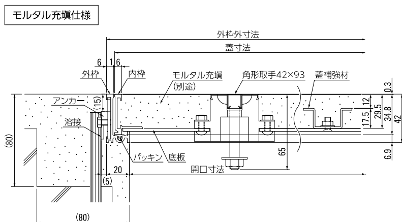
納まり図
