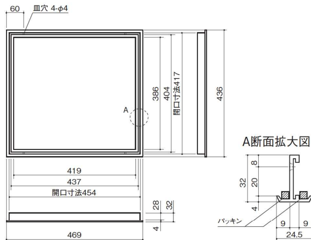
■仕様図(TT-4145P)
