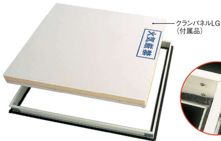
■取付図
