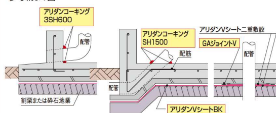
参考納まり図
